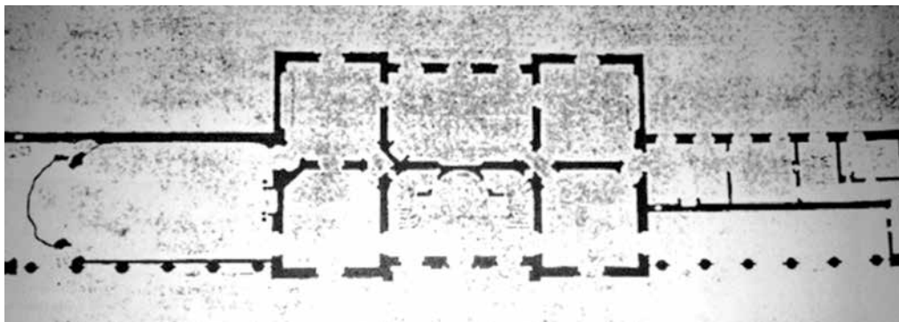
Šeduvos rūmų projekto, kurį parengė architektas Janas Kristianas Kemzeceris (Jan Christian Kemasetzer), pirmo aukšto planas
